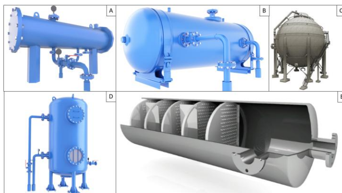
Fig. 1 / 1.1 – Tipuri de recipiente sub presiune: A - Separator orizontal sub presiune; B - Recipient orizontal sub presiune; C - Rezervor sferic sub presiune; D - Separator vertical sub presiune; E - Vas sub presiune cu compartimente interne [1/1, 3/7]
