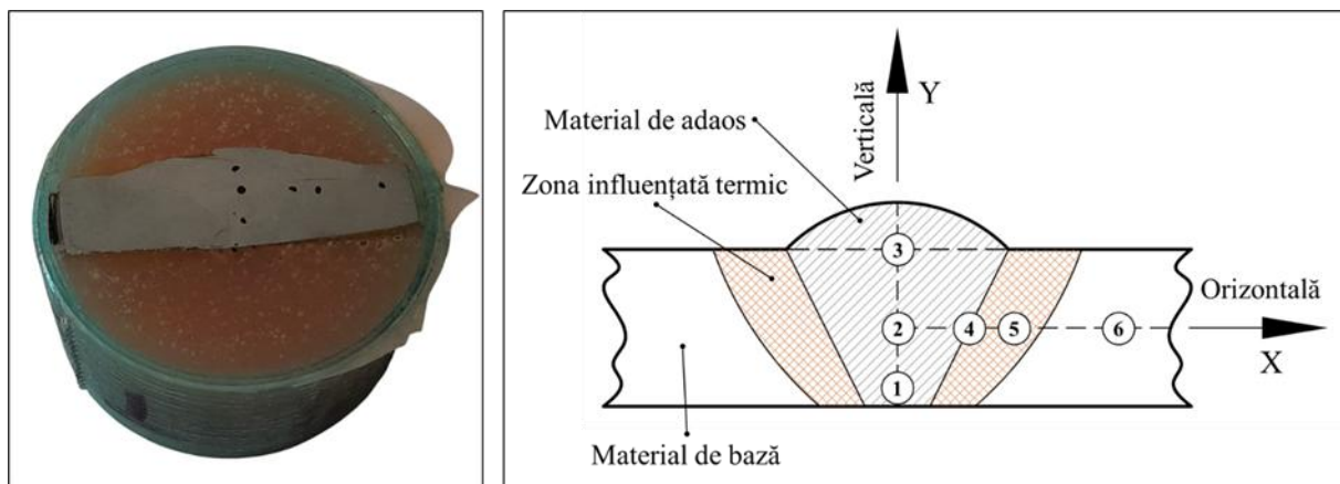
Figura 9/4.7. Proba prelevată pentru testarea durității Vickers (HV) și poziția punctelor în care au fost realizate măsurătorile.
