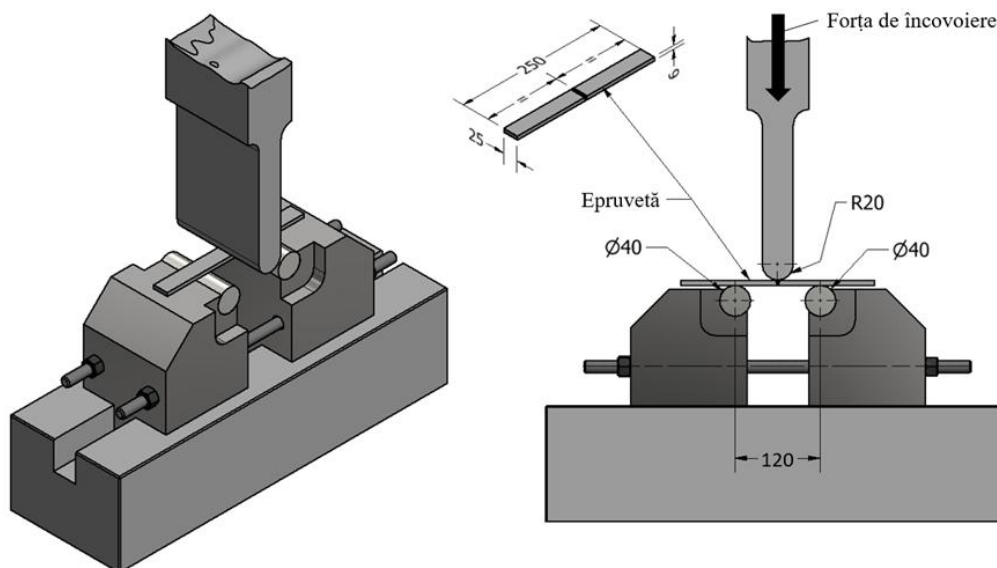
Figura 7/4.5. Schema dispozitivului de fixare a epruvetei de testare la încovoire
