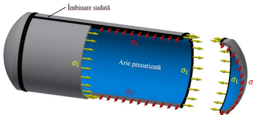
Fig. 2 / 1.2 – Reprezentarea tensiunilor în pereții vaselor cu pereți subțiri
