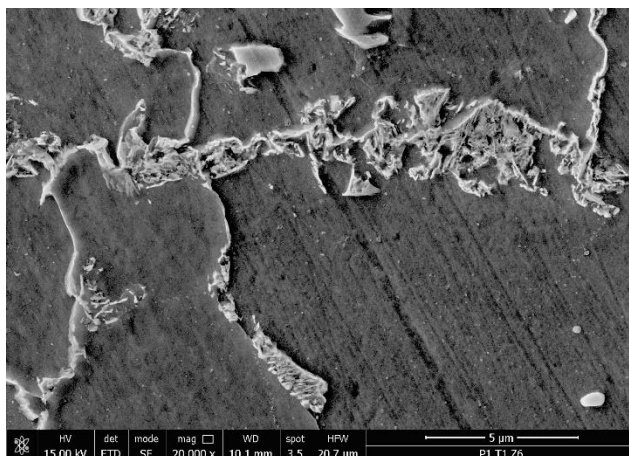
Figura 22/6.8. Structura granulară detaliată a materialului P355N observată la mărirea x20000
