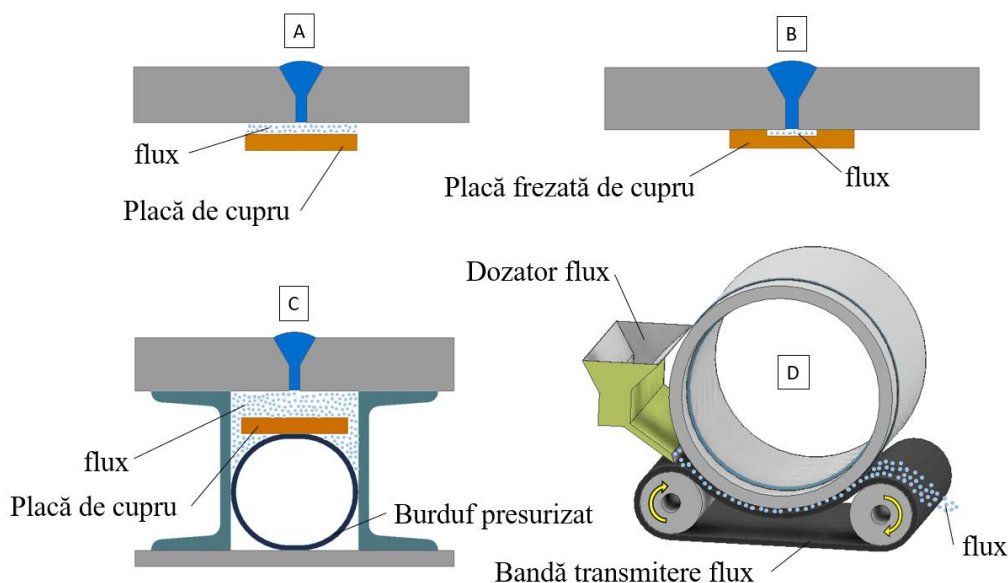
Figura. 3/2.7 – Schema echipamentului de sudare sub strat de flux [8/33]
